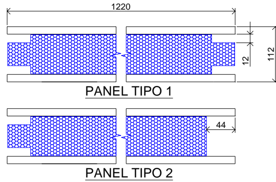
Fig. 3 Terminación lateral de paneles.
