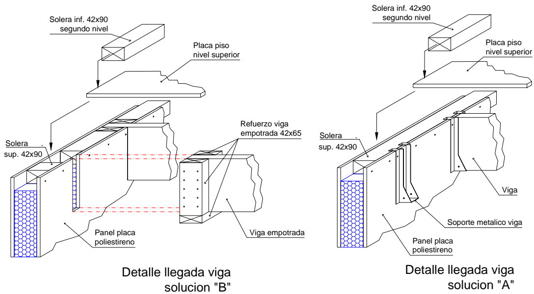
Fig. 5 Llegada viga-panel.
