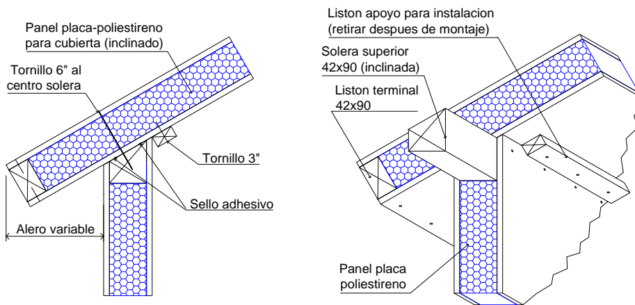
Detalle llegada panel cubierta inclinado
