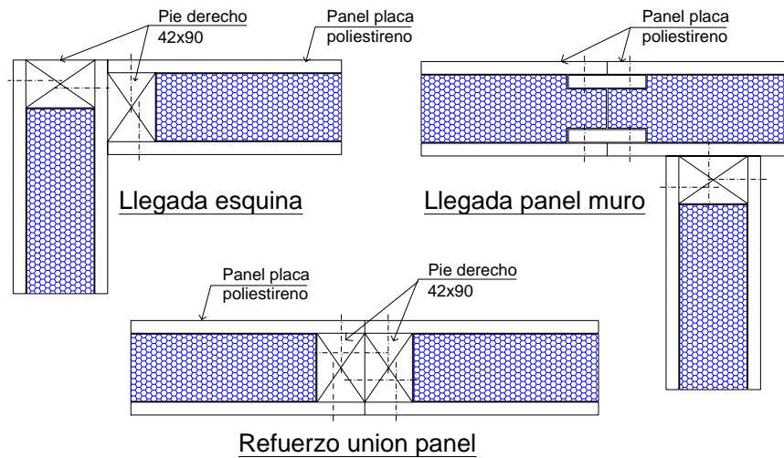
Fig. 4 Unión paneles.
