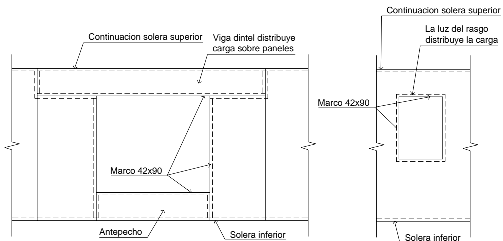
Solucion ventanas
